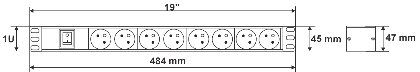
plug: type: E/F („Unischuko”)
